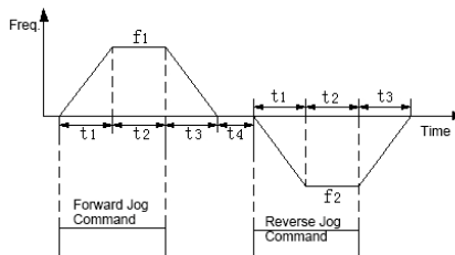
Fig. F8-1 Jog Run
